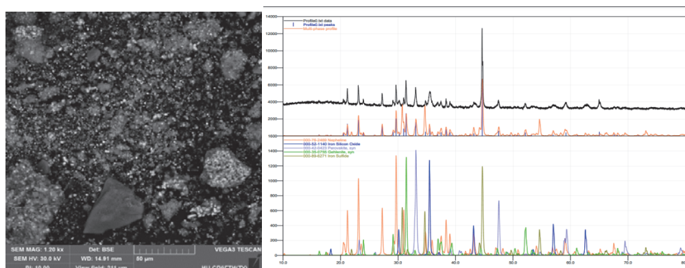
Рисунки 5, 6 – Структура, анализ фаз и состава образца № 2
